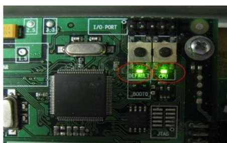
Рис.А.1. Индикаторы DEFAULT и CPU – коммутаторы PSW
