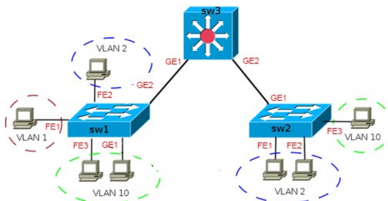
Рис. 5.3.14.1 Топология сети
